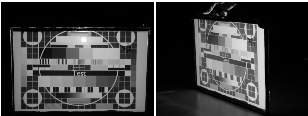
Bild 5. Das Abstrahl- und Diffusionsverhalten des elektrischen schaltbaren Glases ( 0^\circ ; 60^\circ ).
