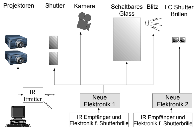
Bild 3. Überblick über das blue-c Gesamtsystem.
